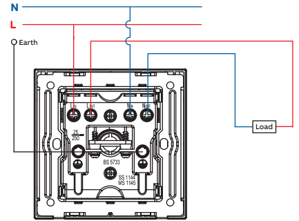
Flex outlet 25A
