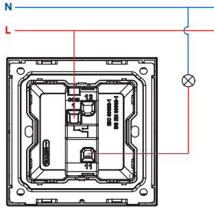
1G 1W switch
