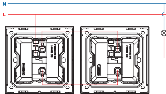
1G 2W switch
