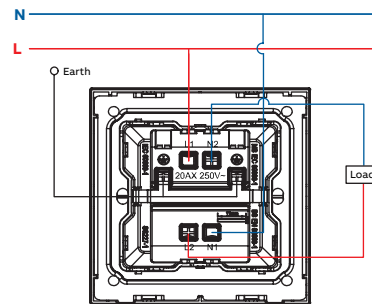
1G 1W switch 20AX DP
