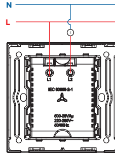
Fan regulator
