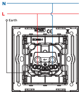
1G 16A SCHUKO Socket
